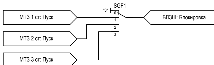
Рисунок 2.4 – Функциональная схема логики БЛЗШ
